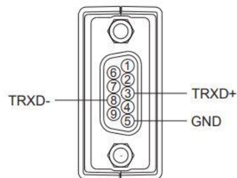
FUS-1D/Combo DB9 Male 커넥터
