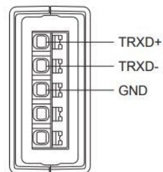
FUS-1T/Combo 터미널블록 커넥터
