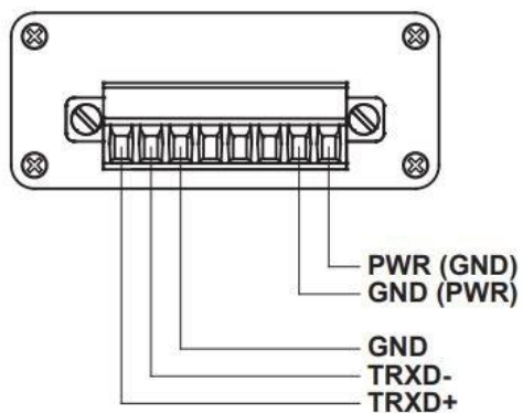
1차측 8핀 터미널블록 커넥터
